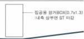
암거box 상세도
