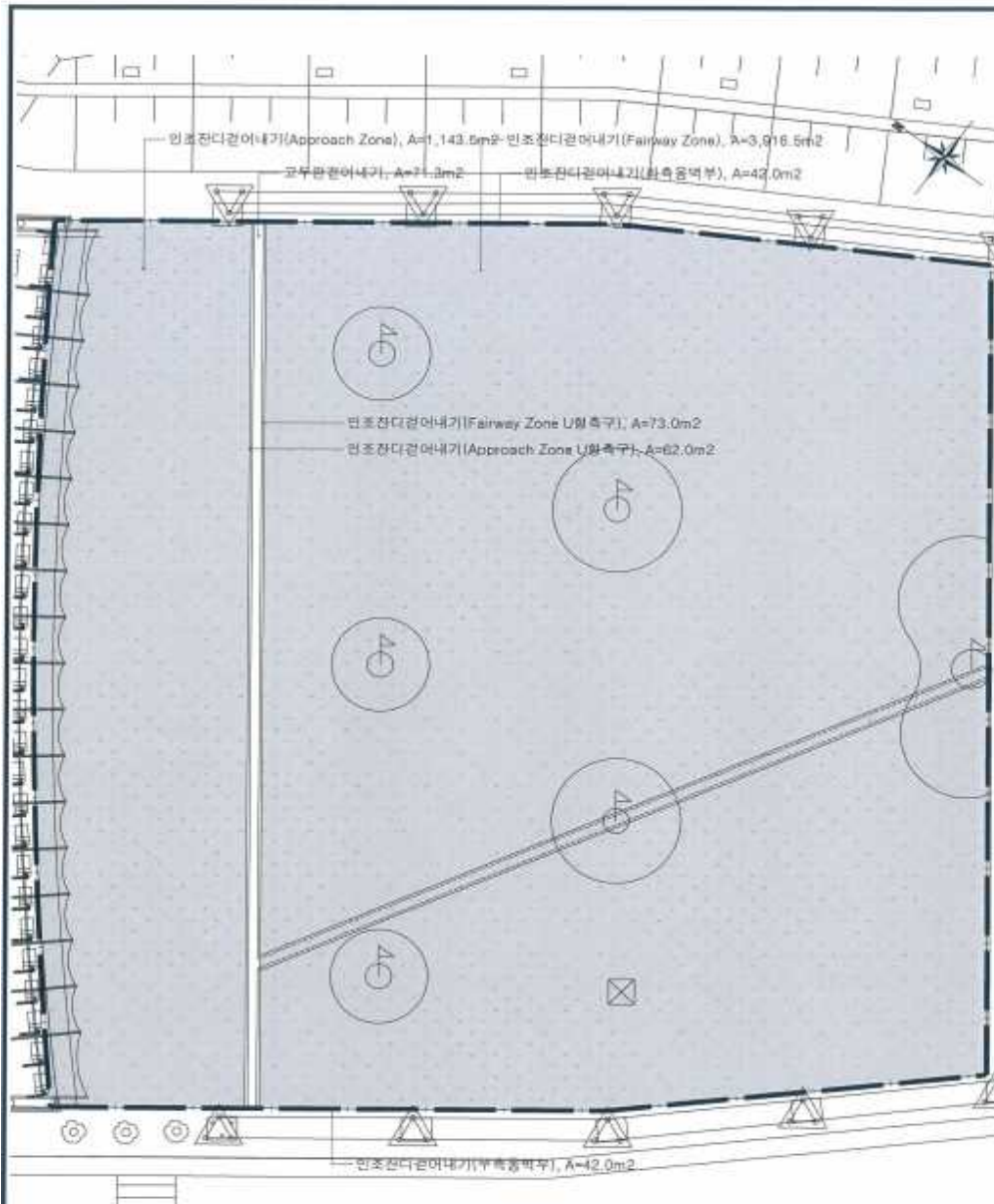
철거 계획평면도 A1-SCALE: 1/200 A3-SCALE: 1/400
