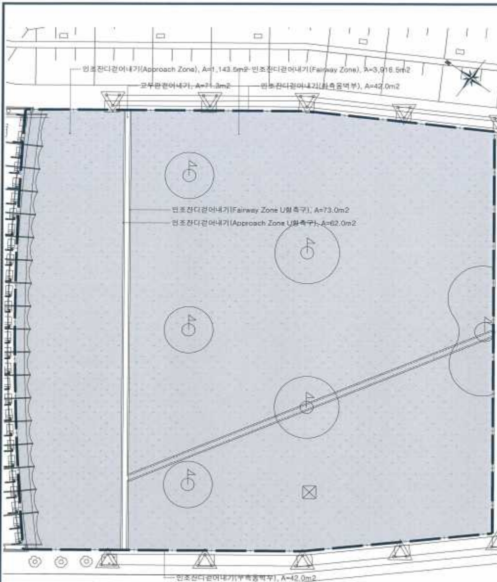
1-1 절거 계획평면도 A1-SCALE 1/200 A3-SCALE 1/400
