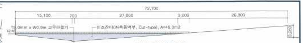
좌측 옹벽부 단면도
