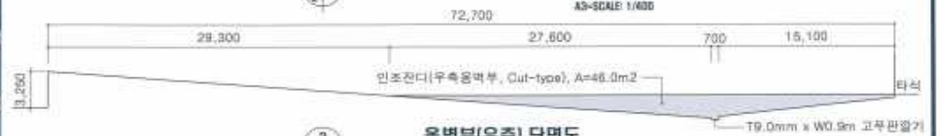
옹벽부(우측) 단면도
