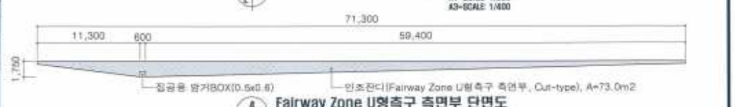
Fairway Zone U형축구 측면부 단면도
