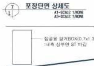
양거box 상세도
